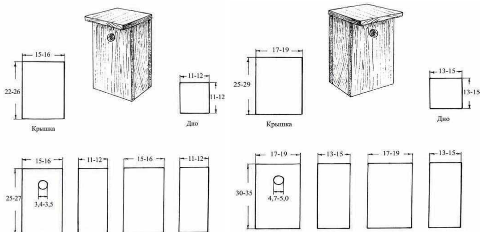
Рис.1 Синичник. Размеры даны из расчета толщины доски 2 см
